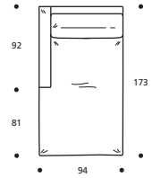
Art. 2113 94 X 173 X h. 88 cm
