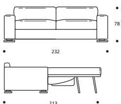
Art. 8853 232 x 92/213 x h. 78 cm
